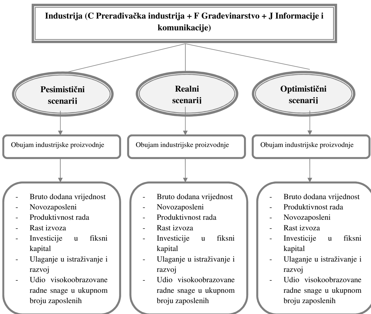
Slika 27. Konceptualni okvir analize scenarija
