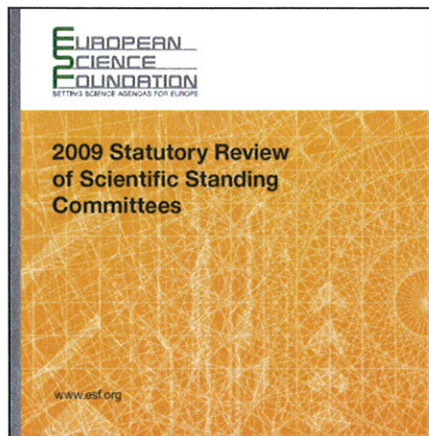
Slika 27. Publikacija 9 donosi rezultate vrednovanja rada Stalnih odbora
