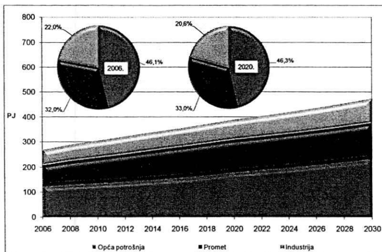
SLIKA 5-2 ODRŽIVI SCENARIJ NEPOSREDNE POTROŠNJE ENERGIJE
