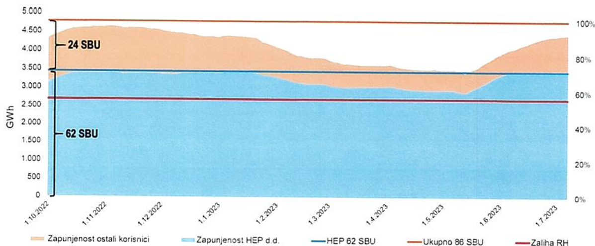
Dijagram 1. Krivulja zapunjenosti PSP u razdoblju od 1. listopada 2022. do 7. srpnja 2023.
